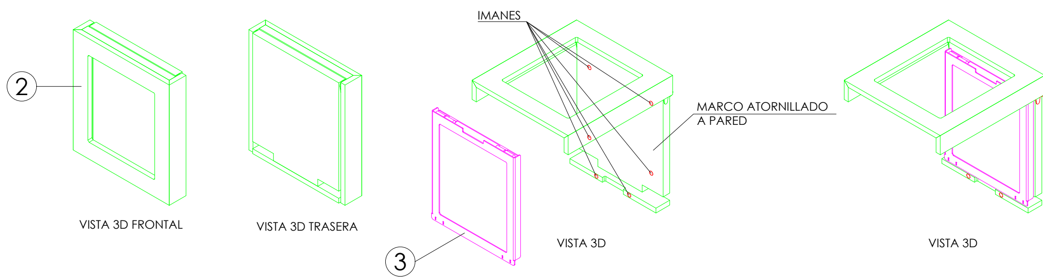
DETALLE MARCO FIJADO A PARED
