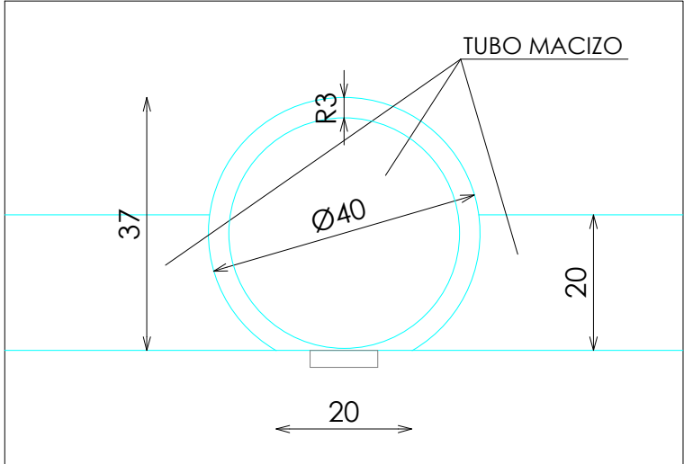
DETALLE D
