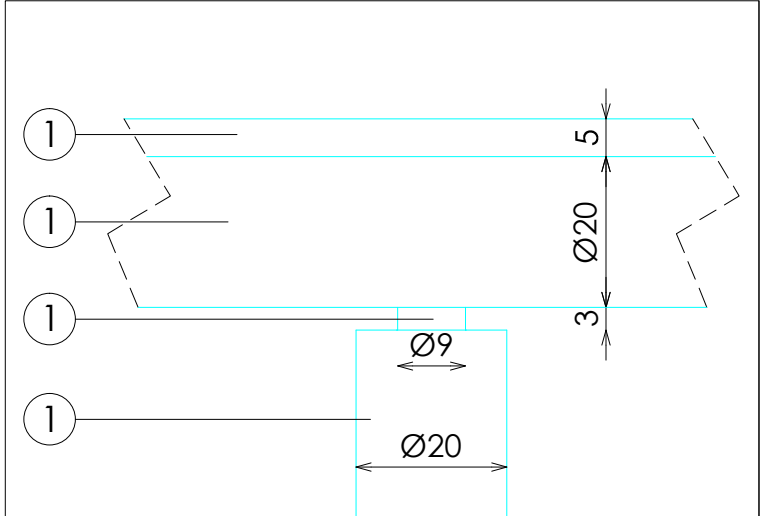
DETALLE B
