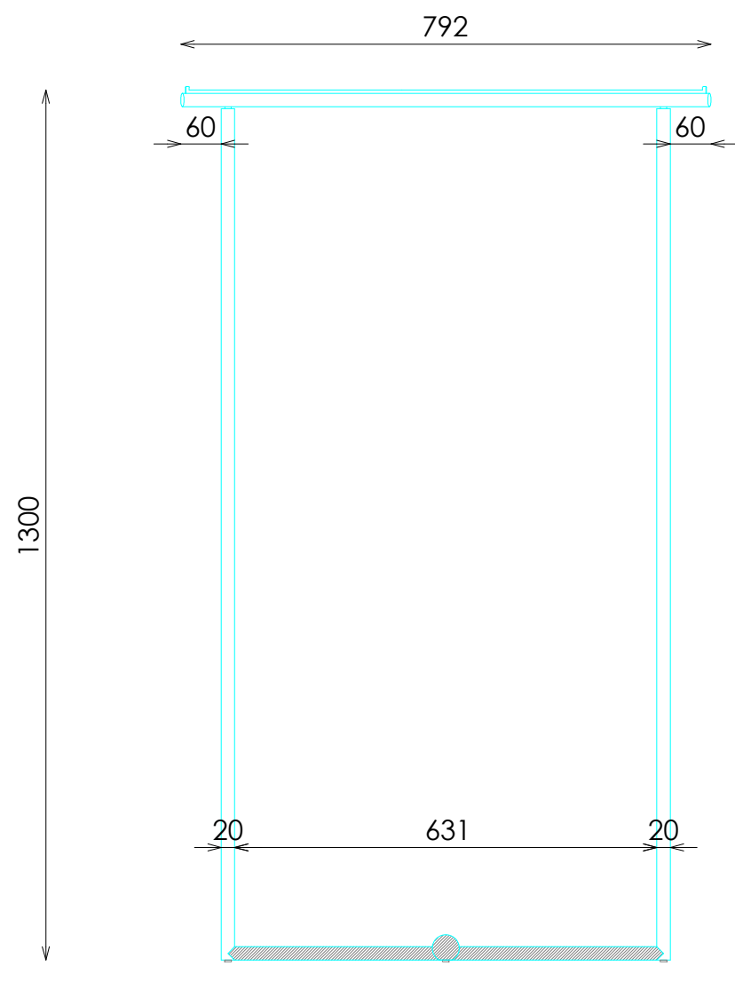
ESTRUCTURA
