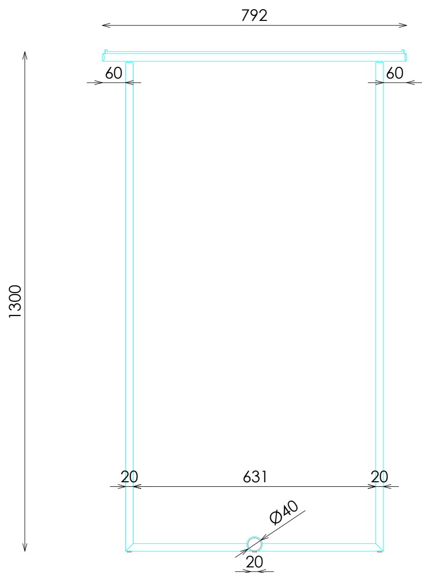
ALZADO
