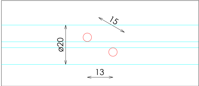
DETALLE D
