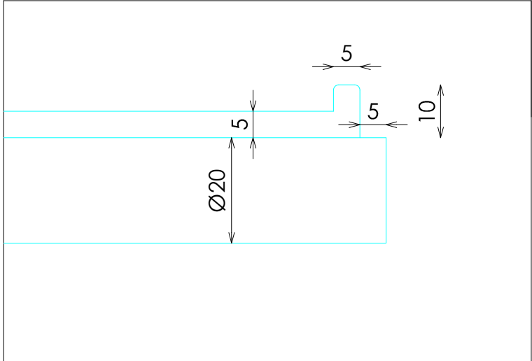
DETALLE C
