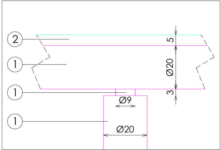
DETALLE B
