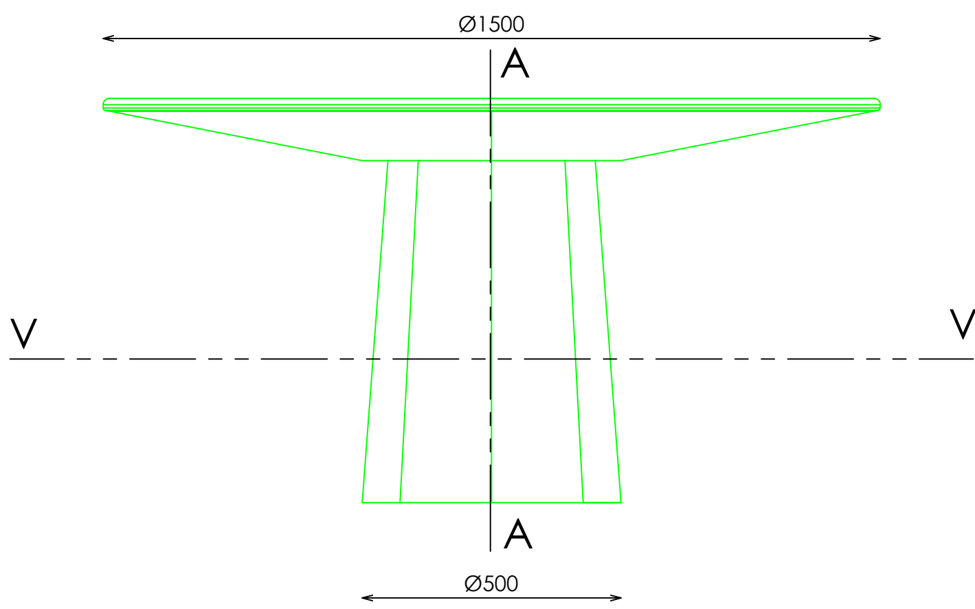
ALZADO
