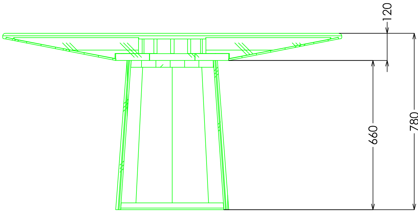
SECCIÓN PERFIL
