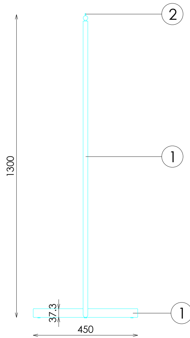
PERFIL
