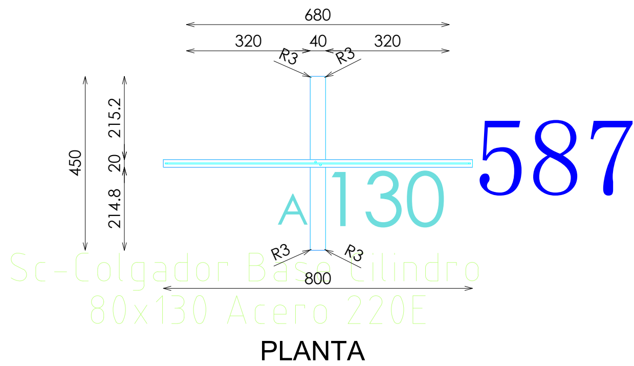
PLANTA
