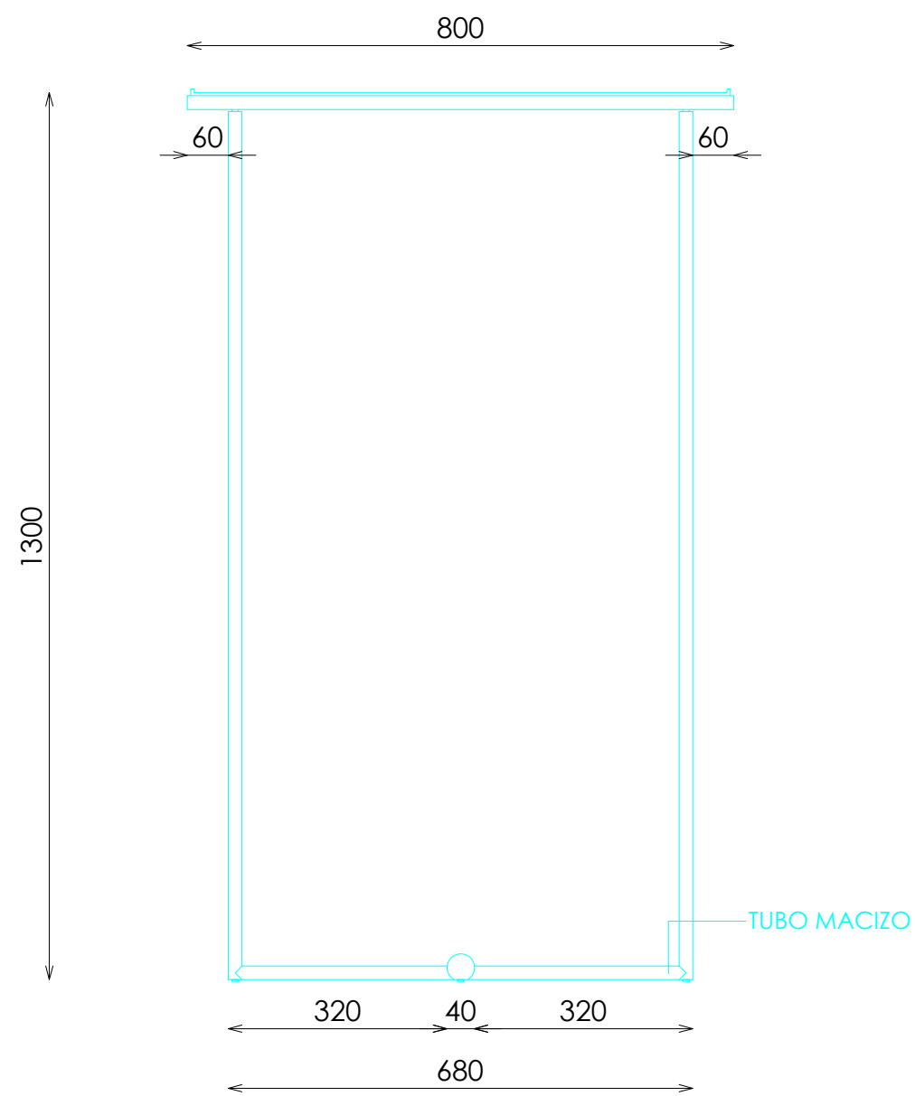
ESTRUCTURA
