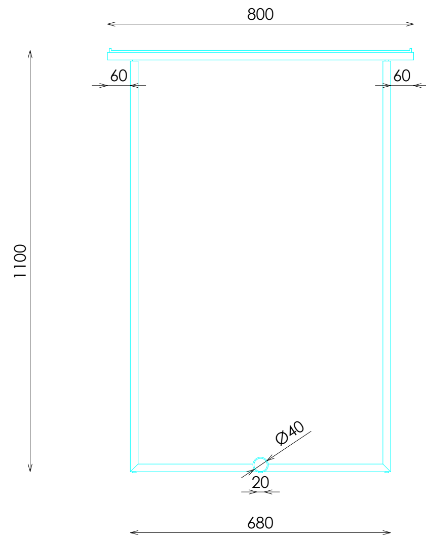
ALZADO
