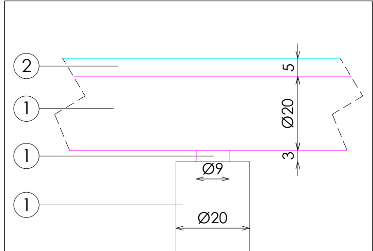
DETALLE B
