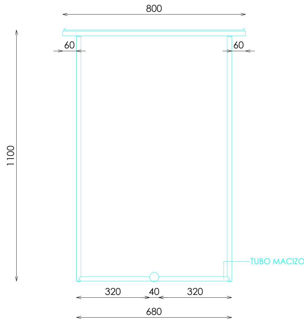
ESTRUCTURA
