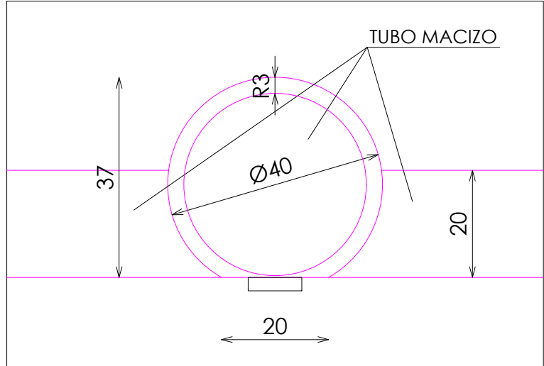
DETALLE D
