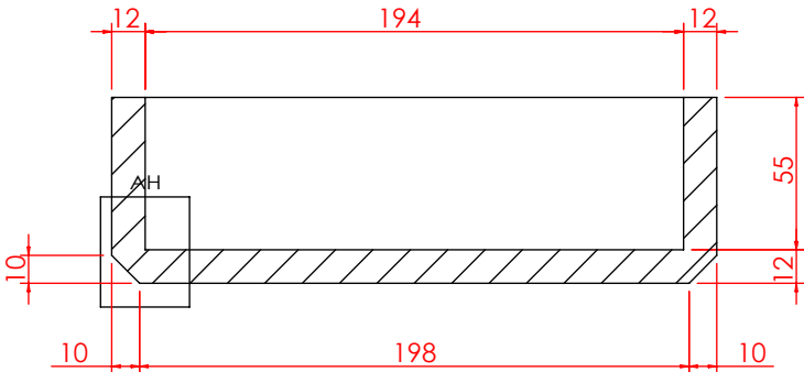
剖面 AG-AG
