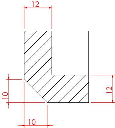
局部视图 AH 比例 1 : 1
