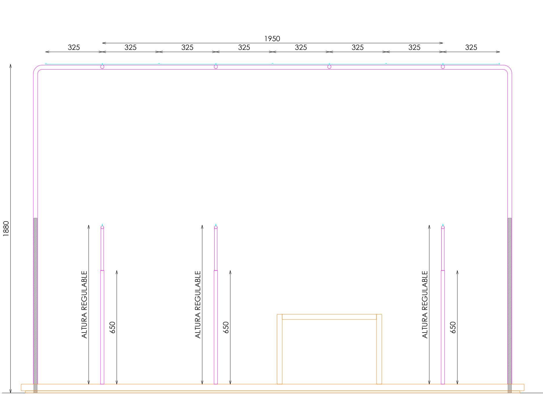
ALZADO FRONTAL
