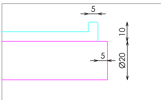
DETALLE ANTIROCE
