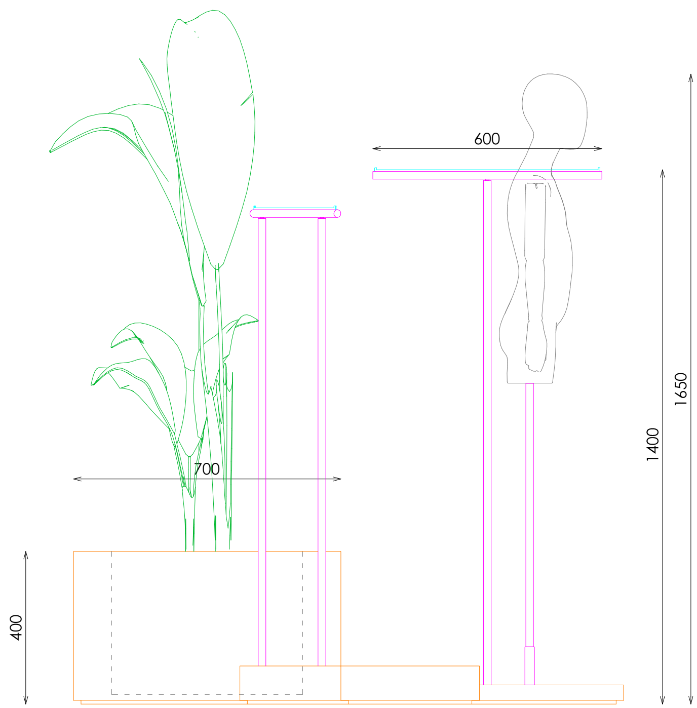
ALZADO LATERAL
