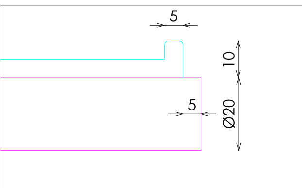
DETALLE ANTIROCE
