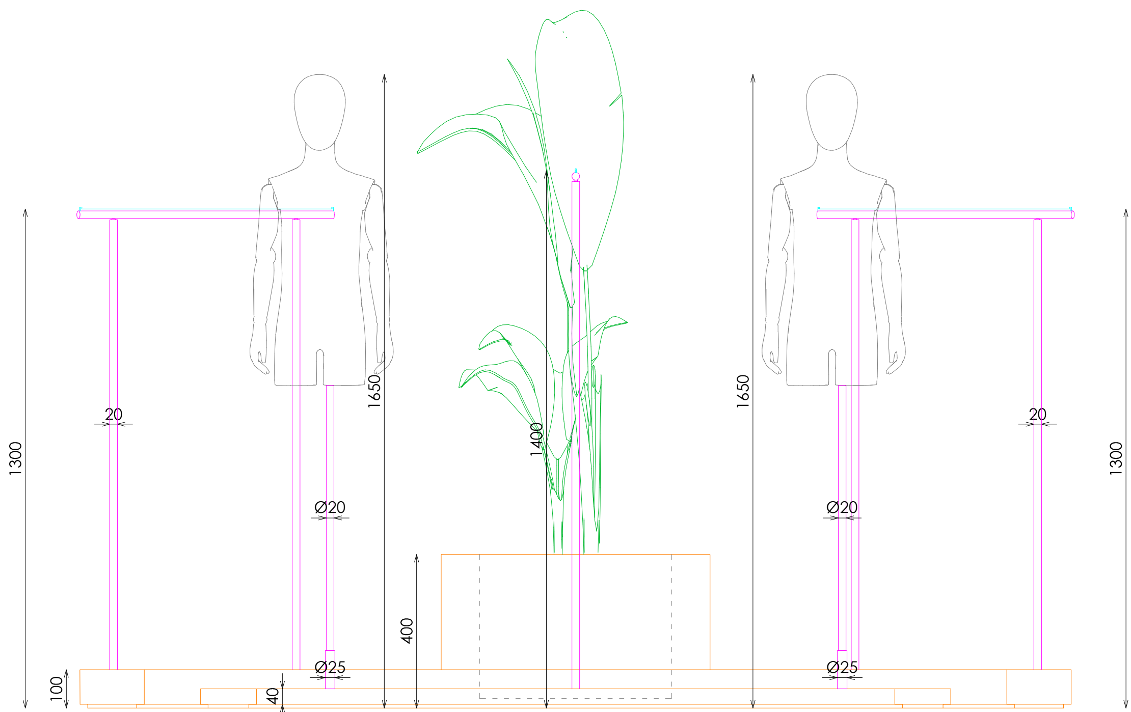
ALZADO FRONTAL
