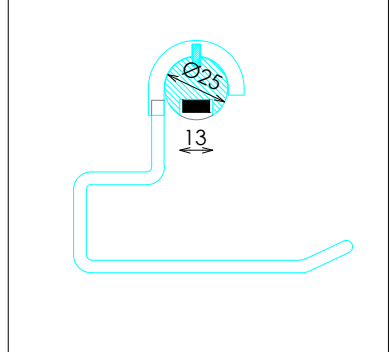
DET. PINCHO COMPL.
