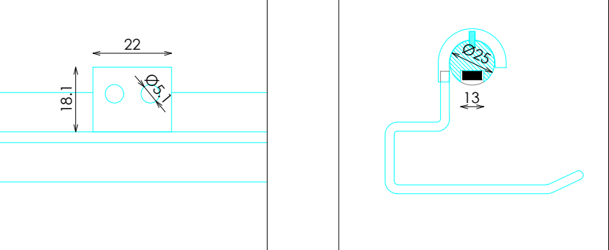
DETALLE FRONTALES EXTRAIBLES
