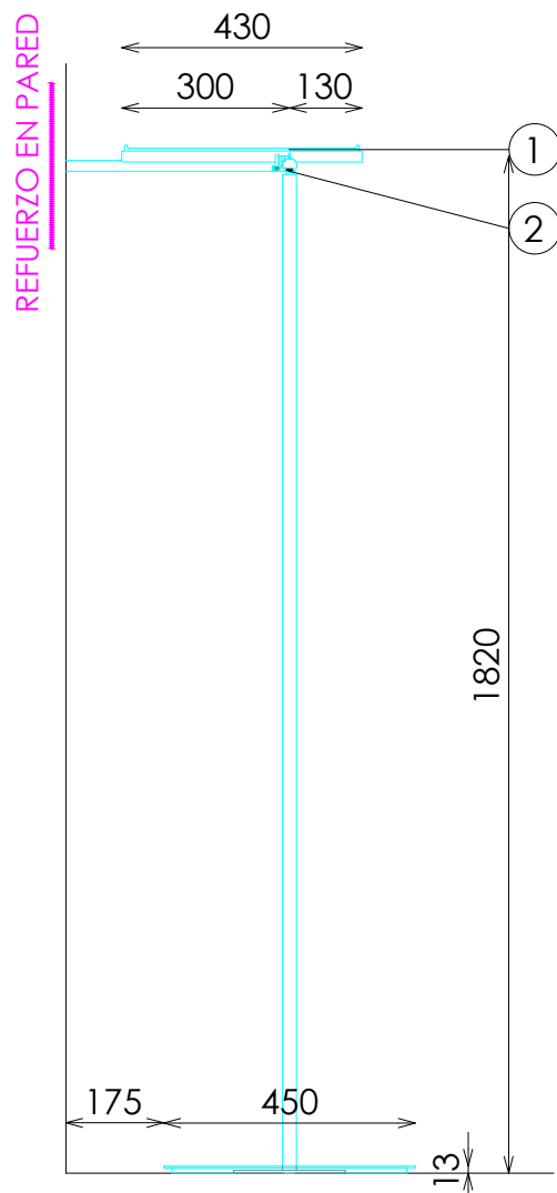
SECCIÓN
