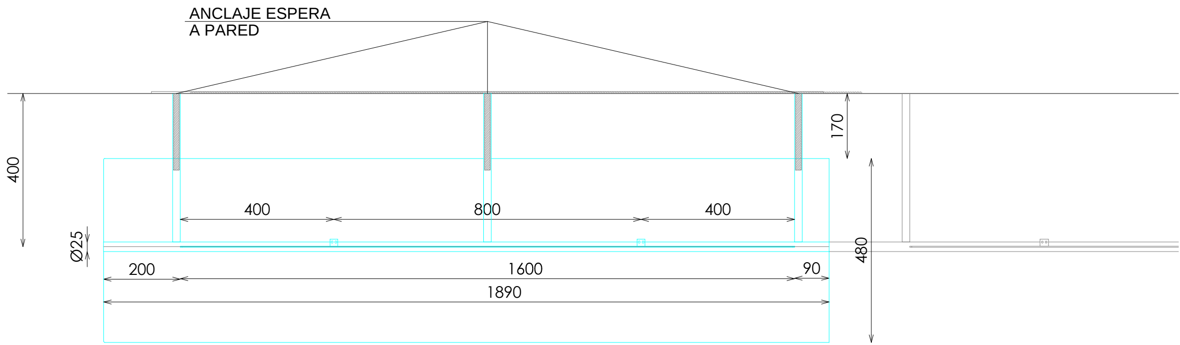
PLANTA
