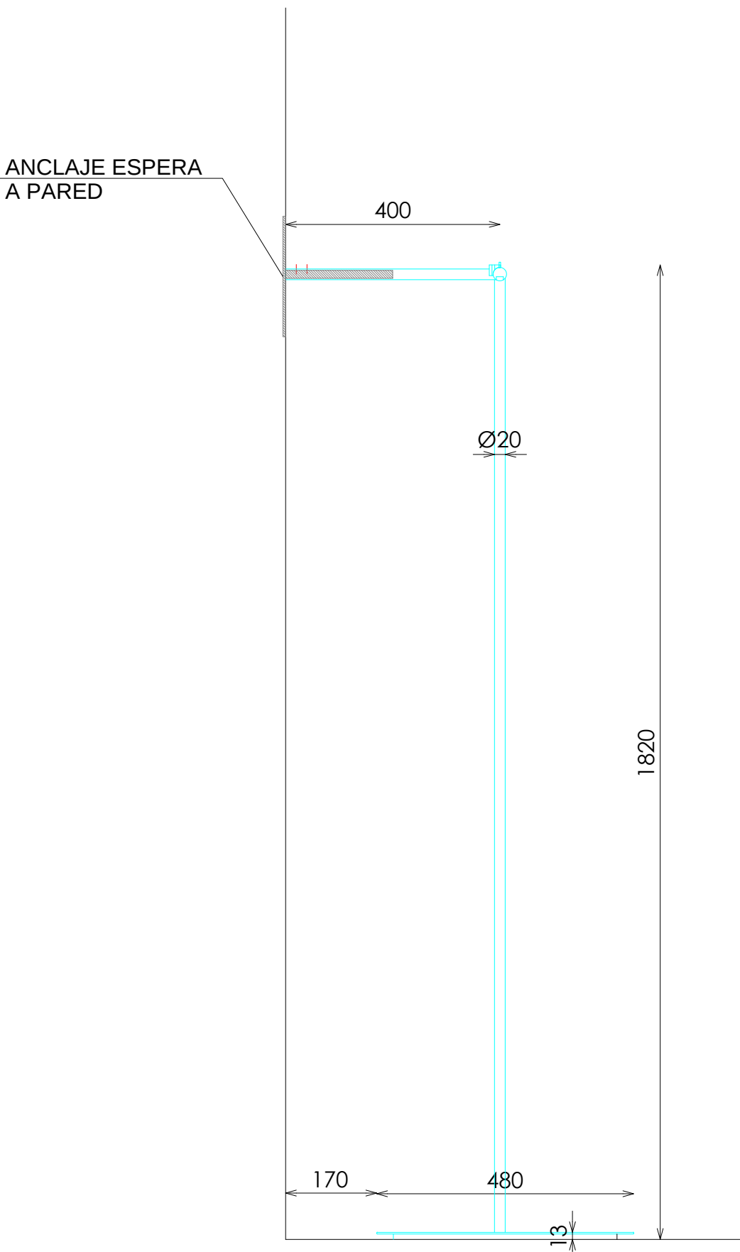
PERFIL SECCIONADO
