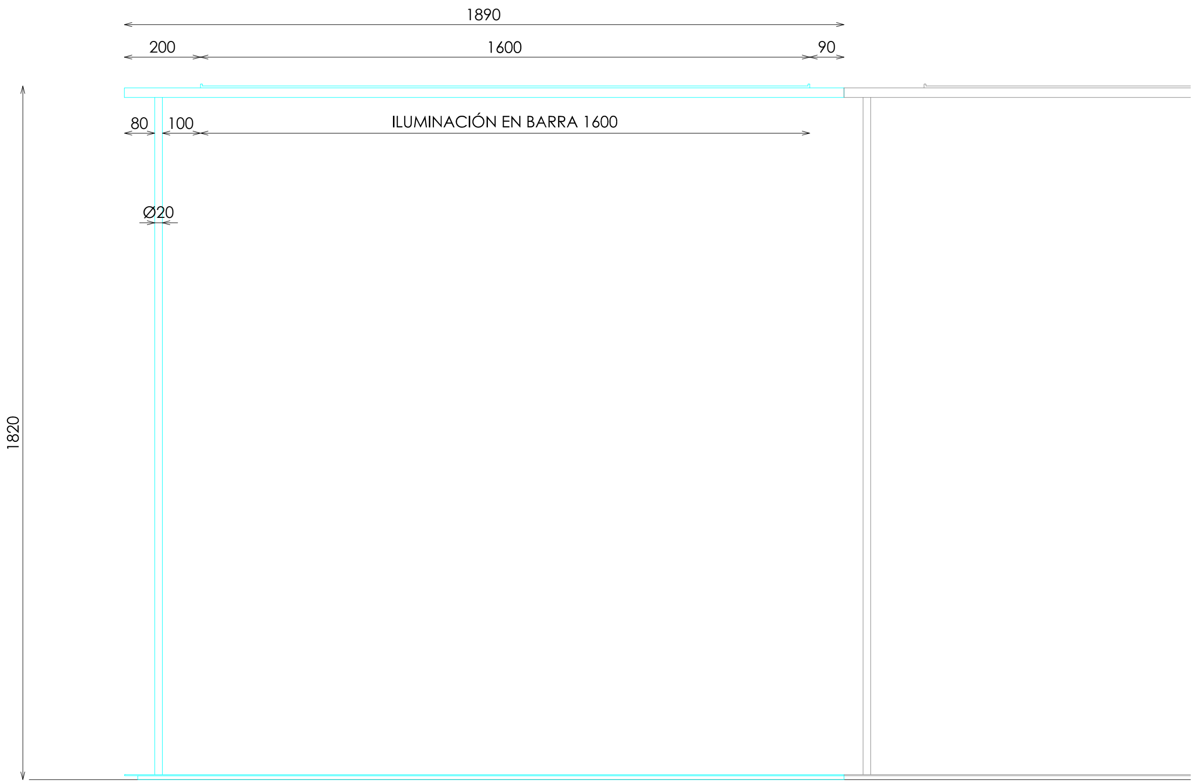
ALZADO FRONTAL
