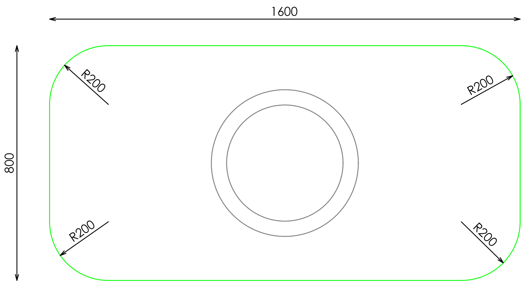
PLANTA
