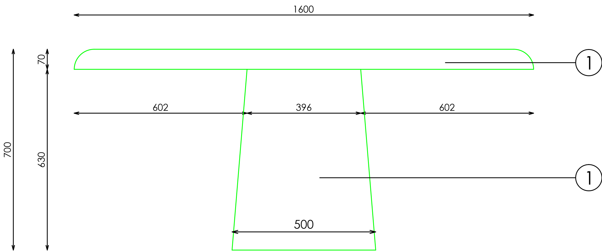
ALZADO
