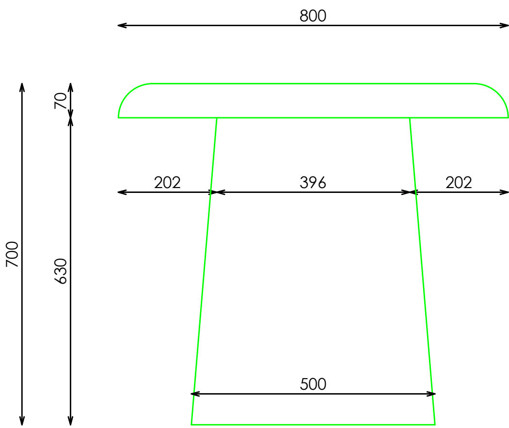
PERFIL
