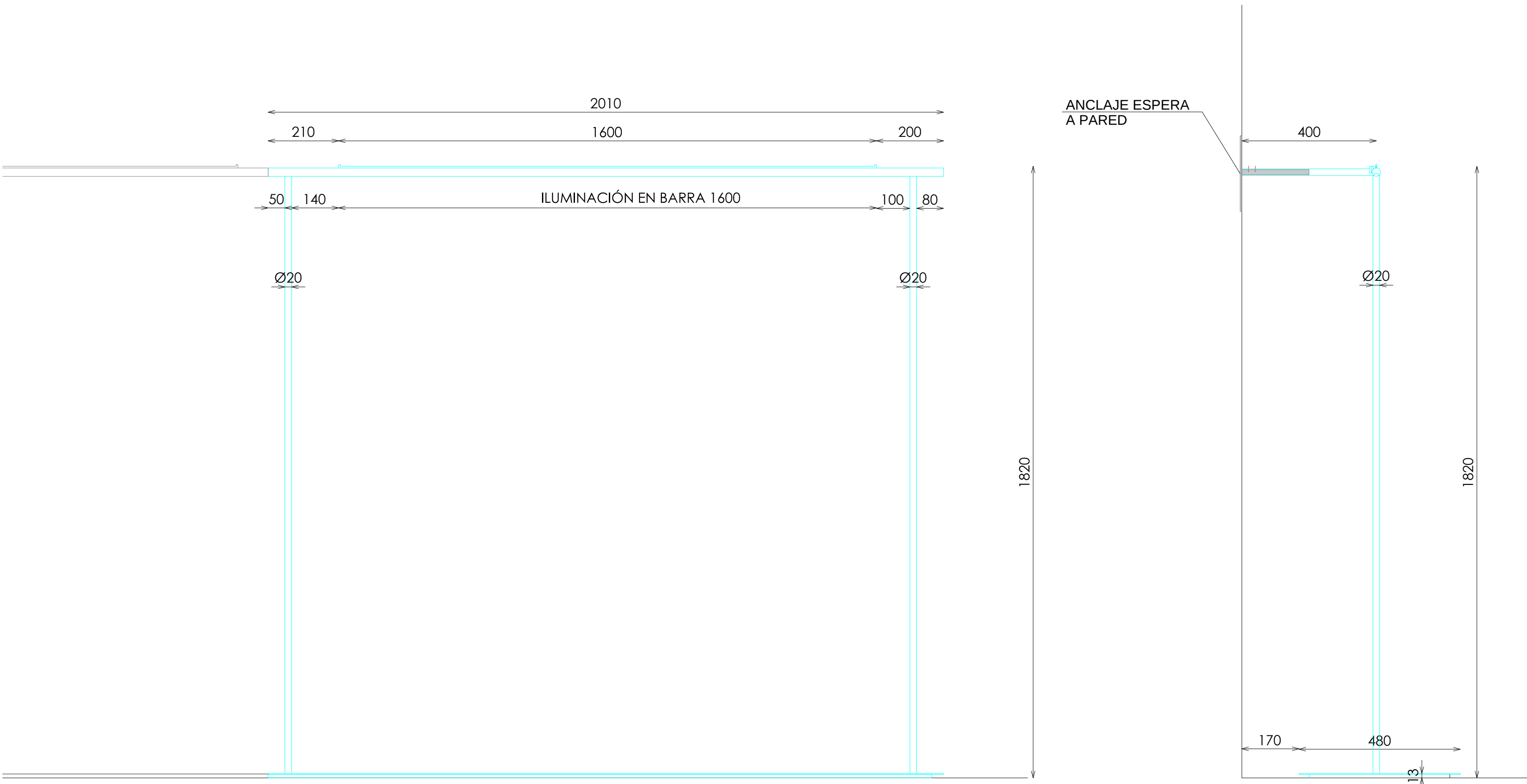
PERFIL SECCIONADO
