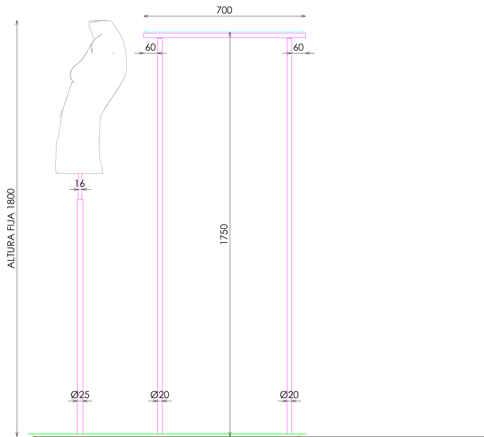
ALZADO LATERAL
