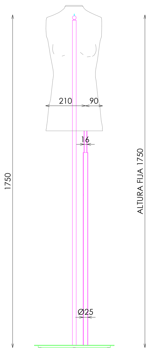
ALZADO FRONTAL
