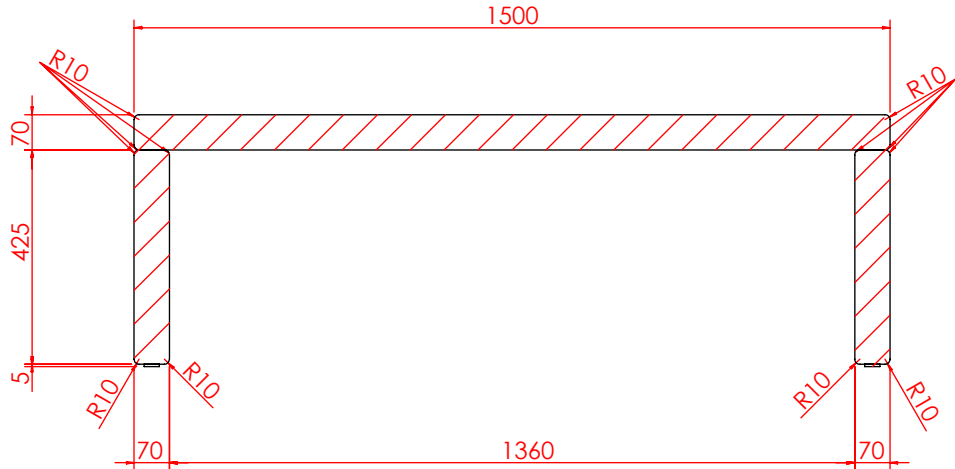
剖面 AG-AG
