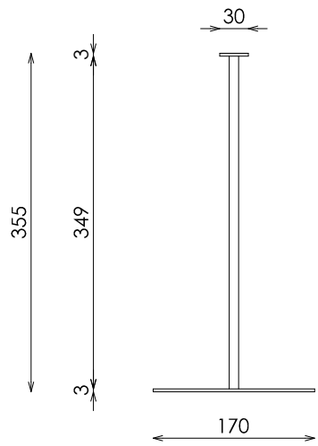
ALZADO
