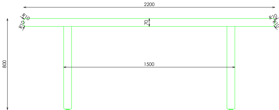
ALZADO
