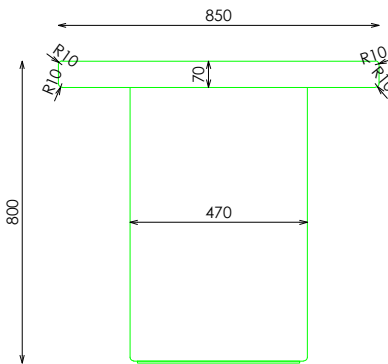
PERFIL
