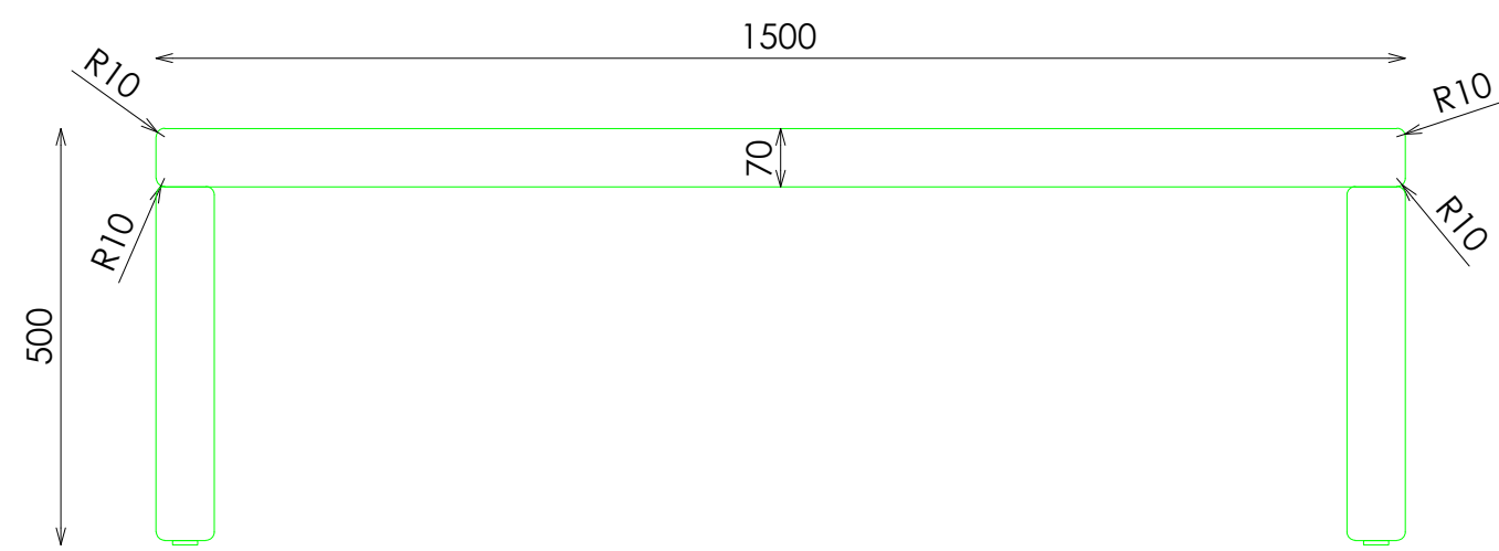
ALZADO
