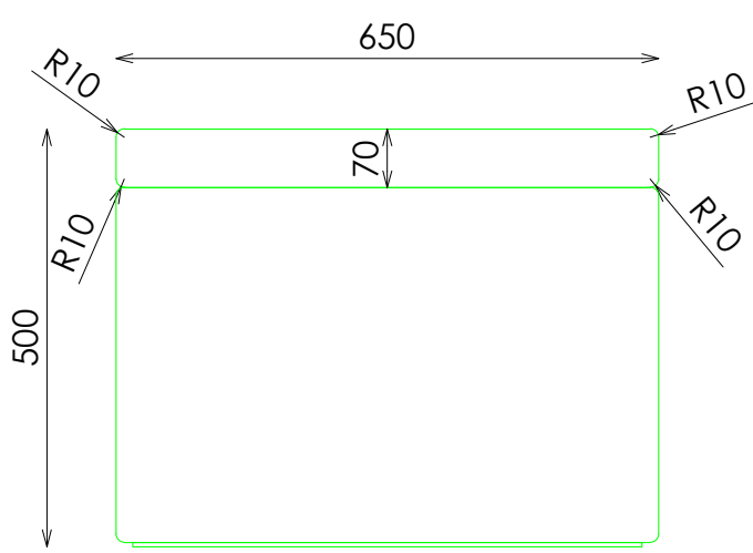
PERFIL
