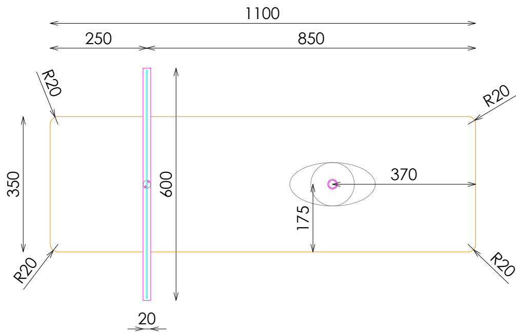
PLANTA
