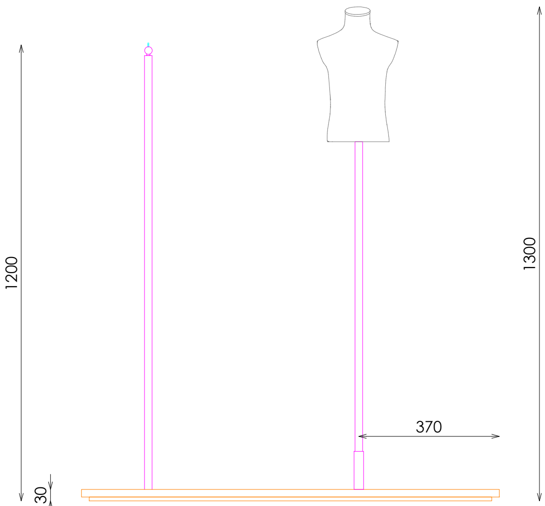
ALZADO
