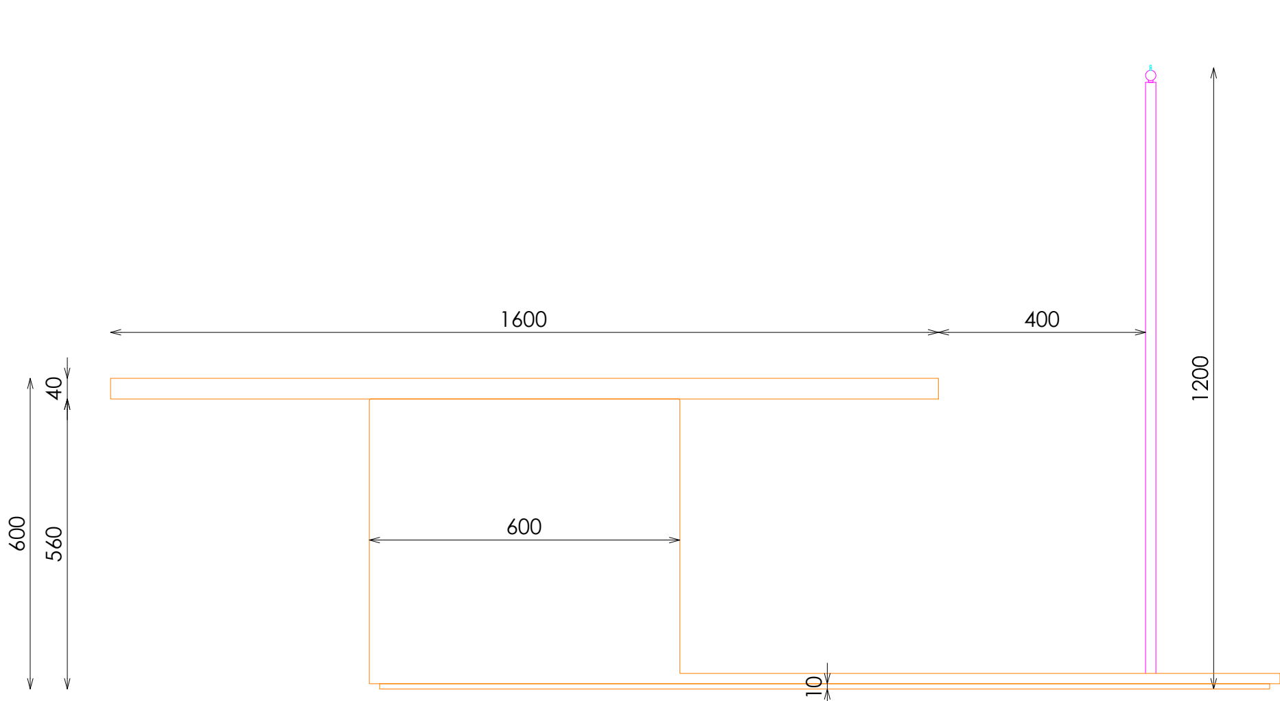
ALZADO
