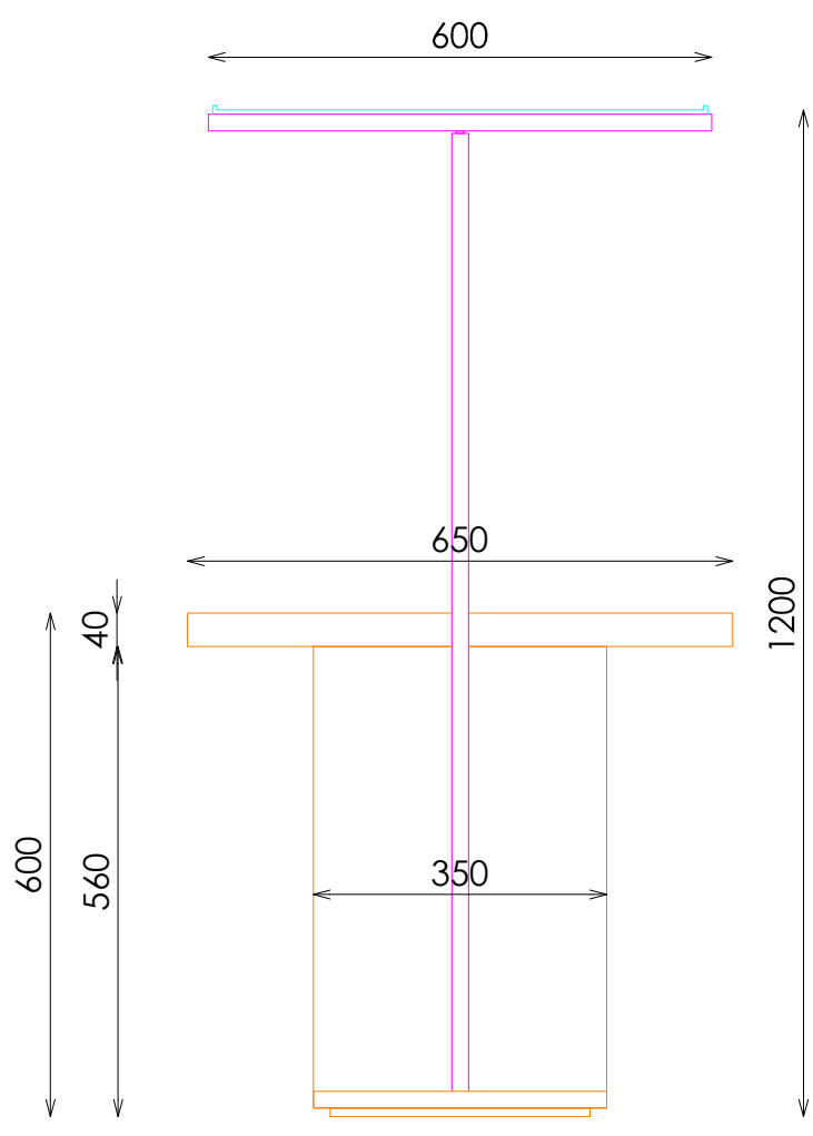
PERFIL DERECHO
