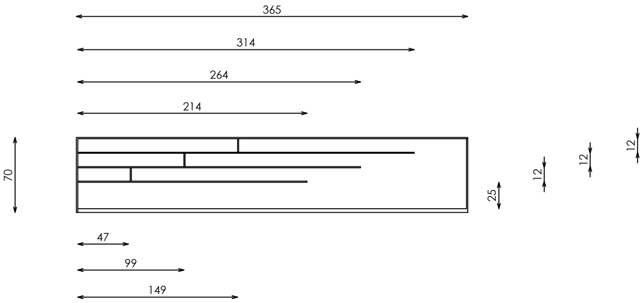
PLANTA
