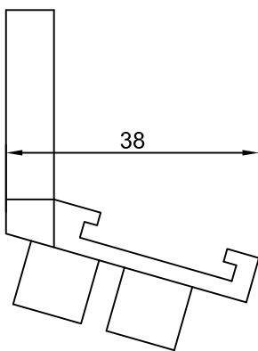
SECCIÓN PERFIL
