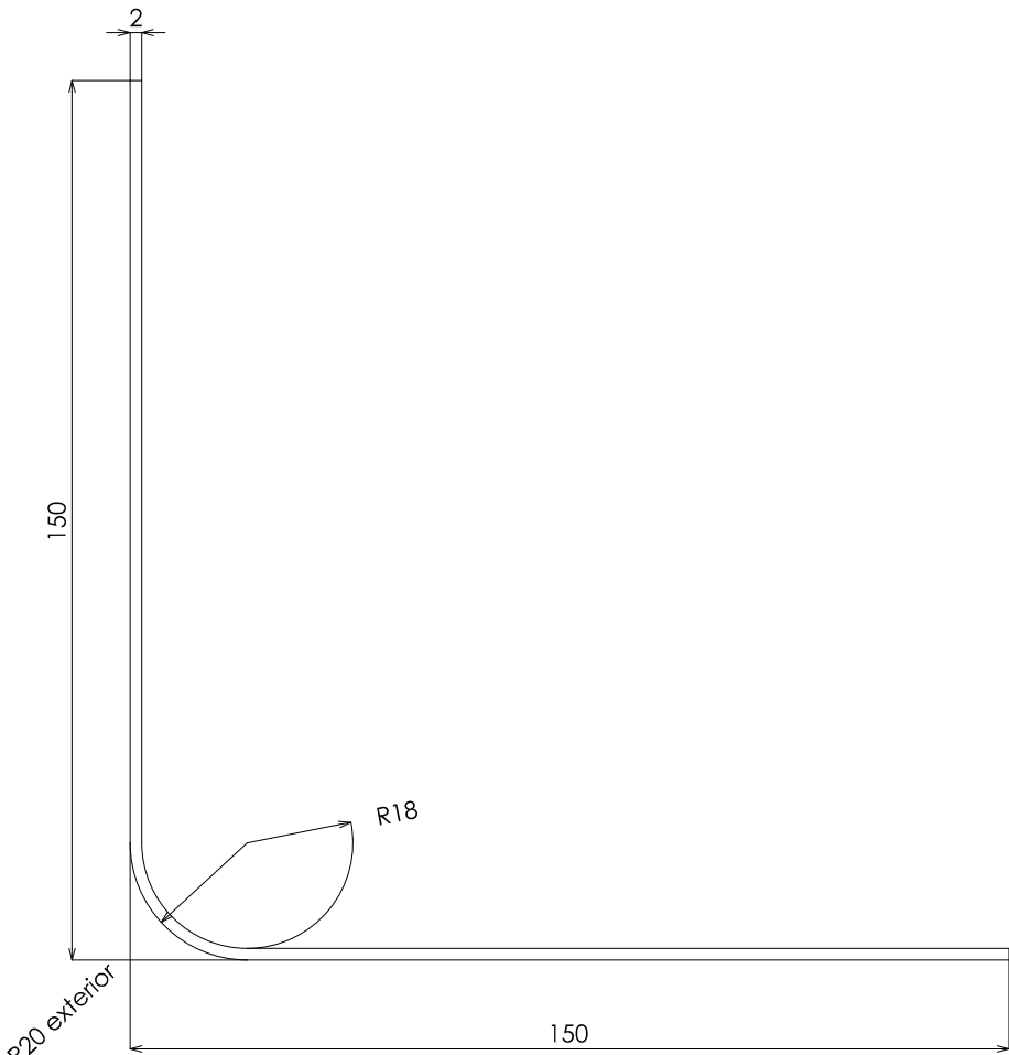
ALZADO
