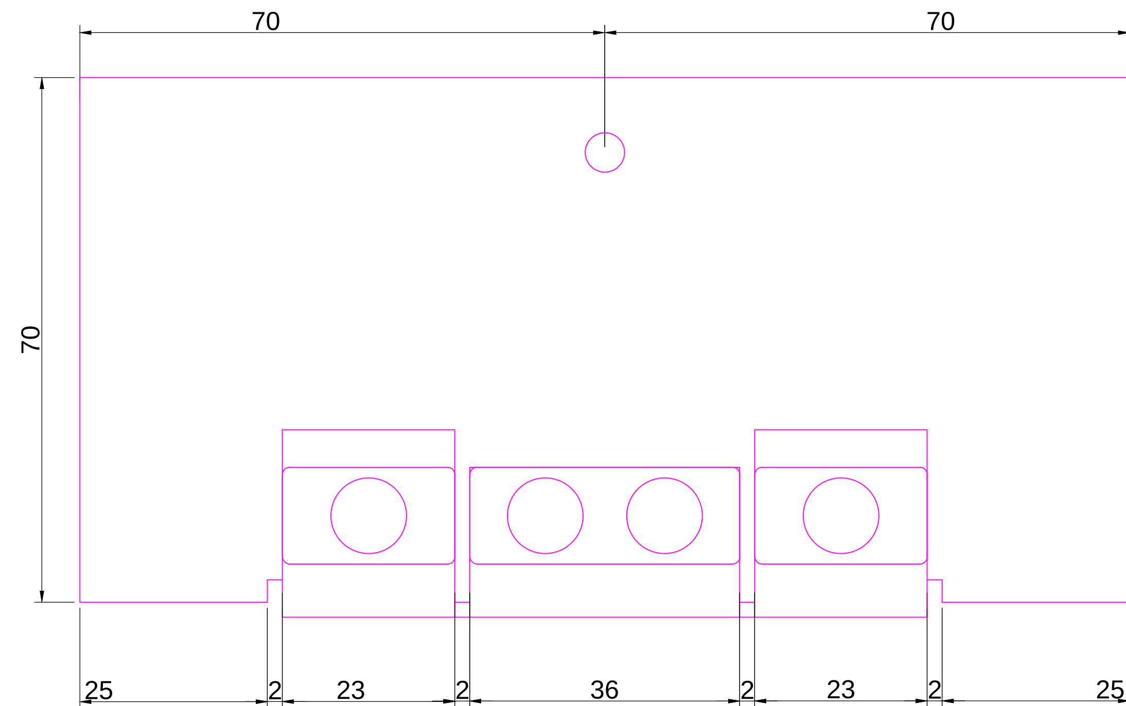
ALZADO
