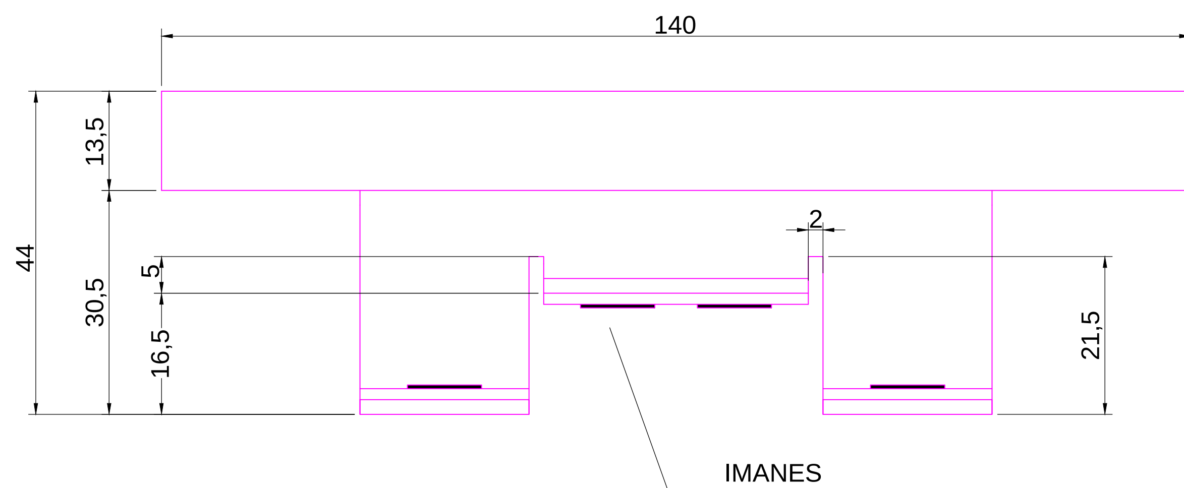
ALZADO
