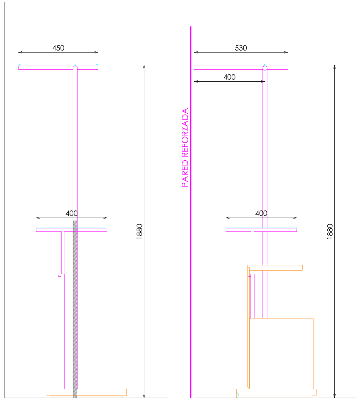
ALZADO LATERAL
