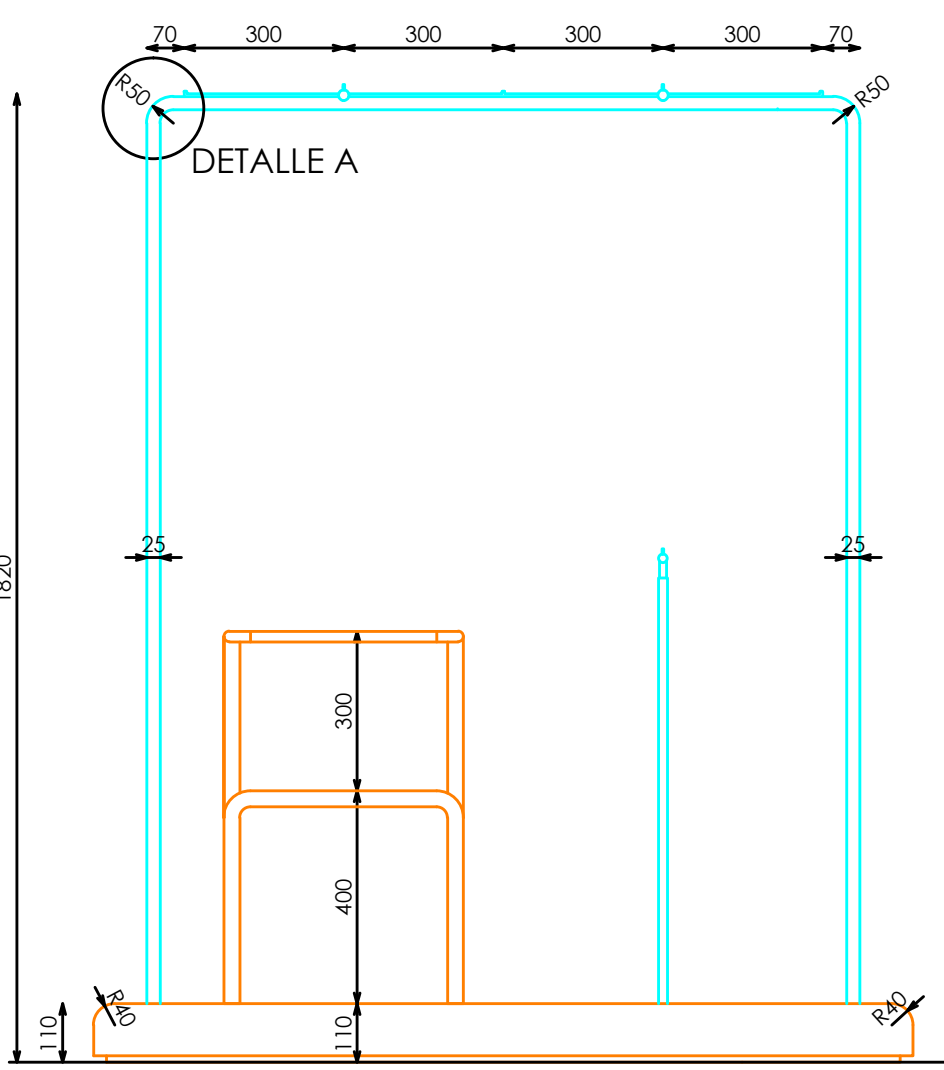
ALZADO FRONTAL
