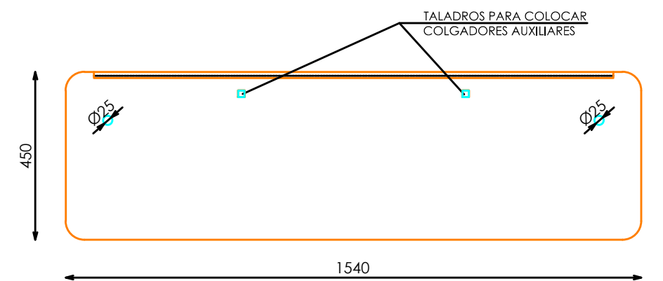
PLANTA SECCIONADA (ILUMINACIÓN EN TARIMA)
