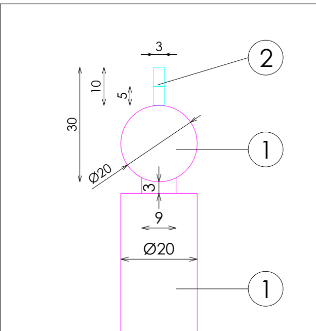
DETALLE ANTIROCE
