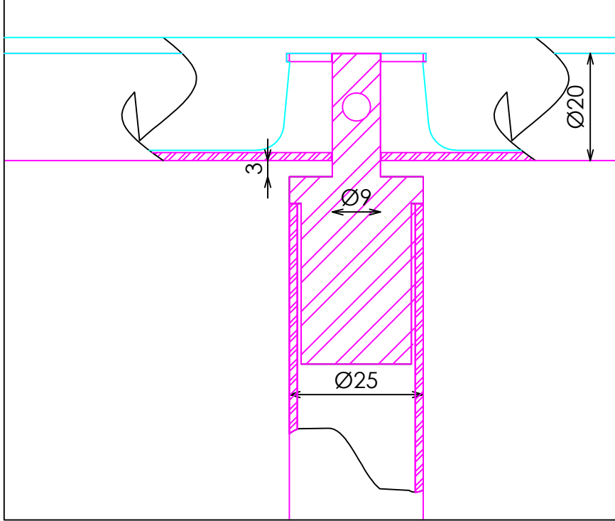
DETALLE C (SECCIÓN)
