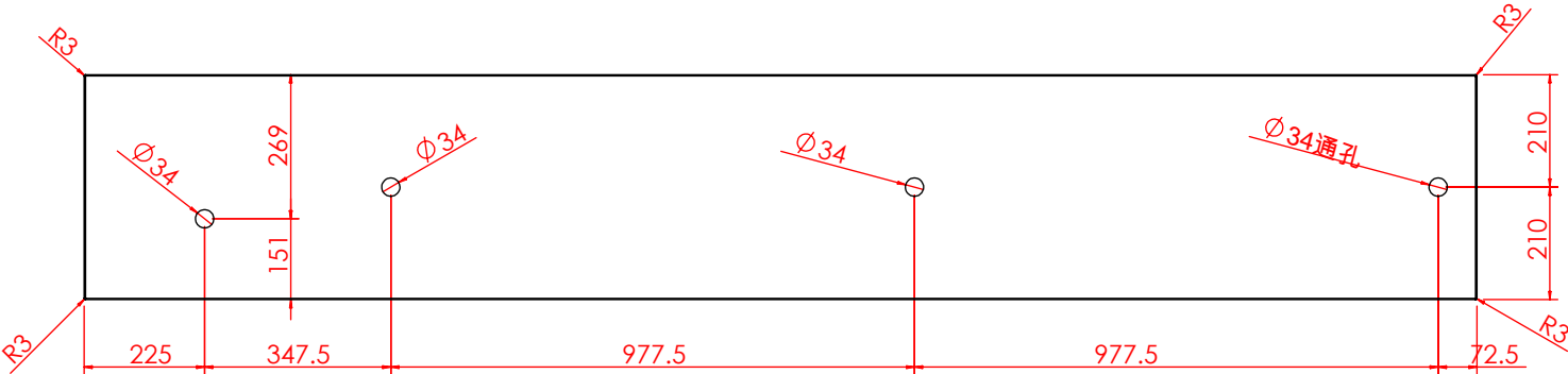
局部视图 AG 比例 2 : 1
