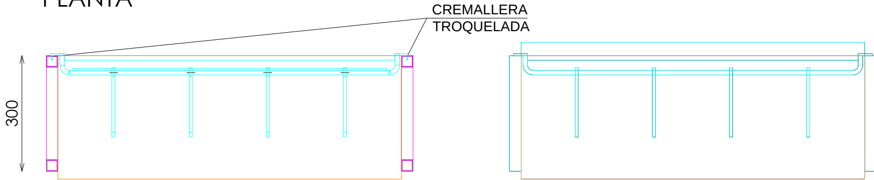
PLANTA SECCIONADA (DOTACIÓN COMPLEMENTOS)
