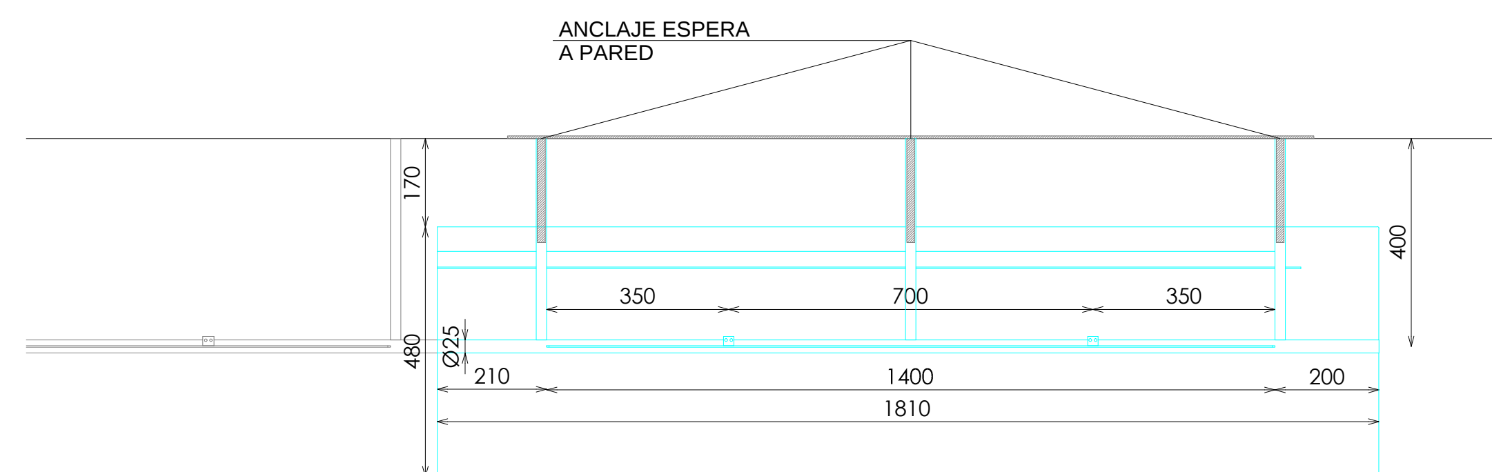
PLANTA
