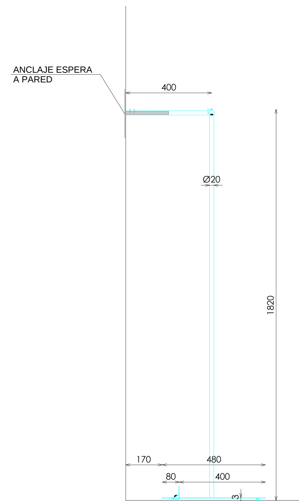
PERFIL SECCIONADO
