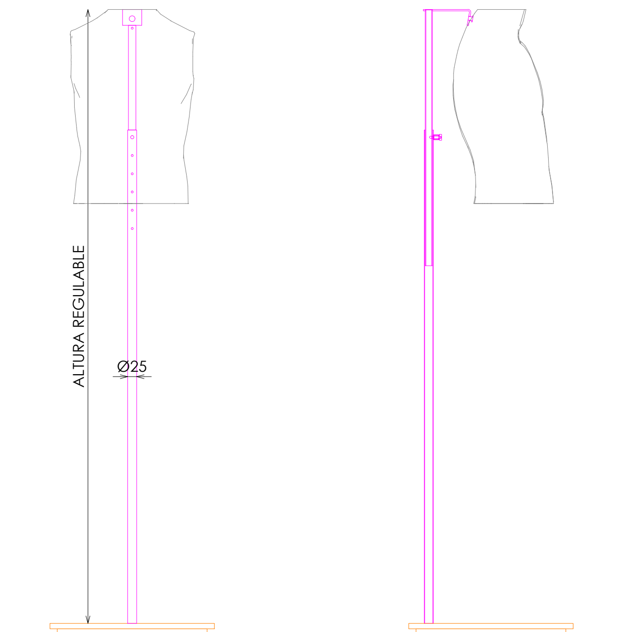
ALZADO
