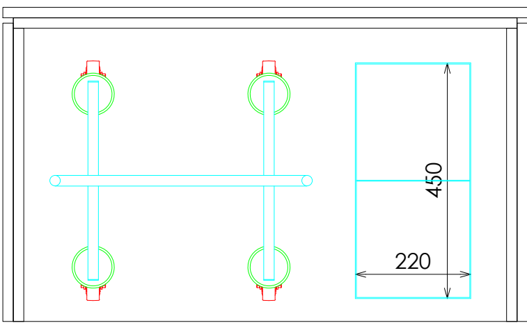
PLANTA SECCIONADA
