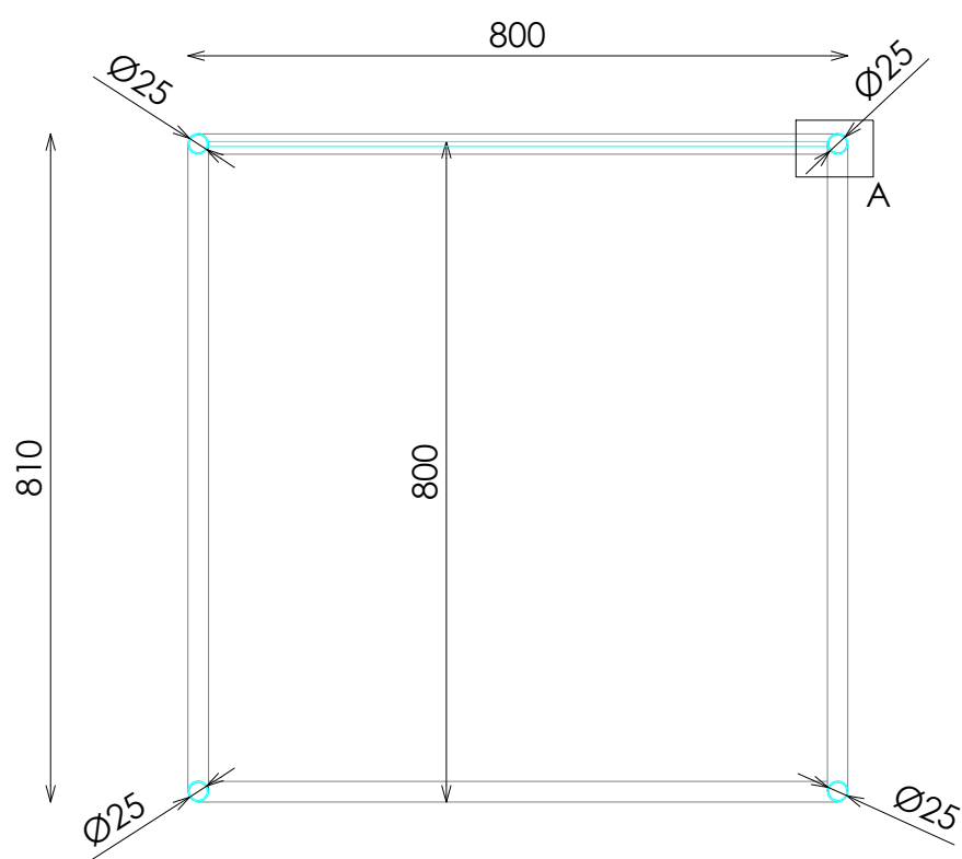
ALZADO SECCIONADO
