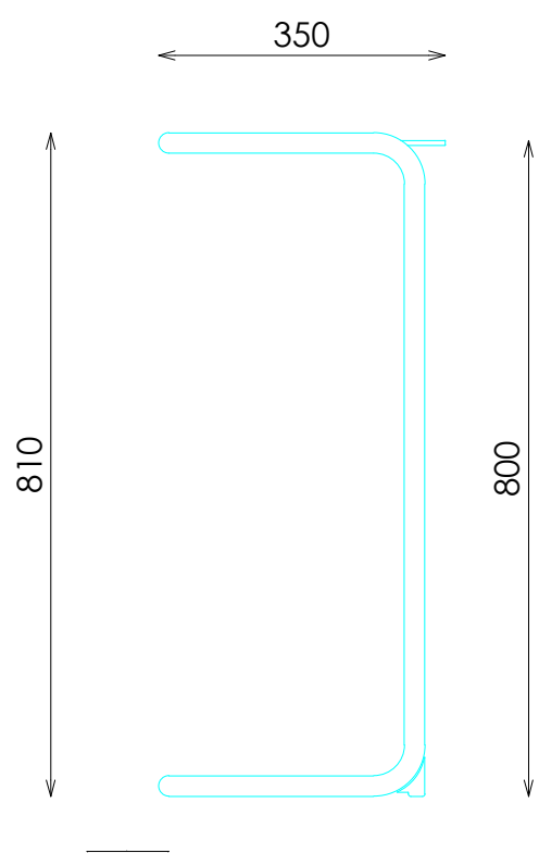
PERFIL
