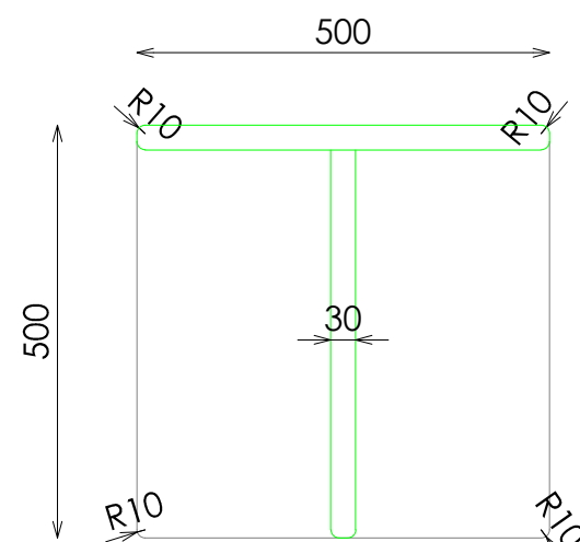
PERFIL SECCIONADO
