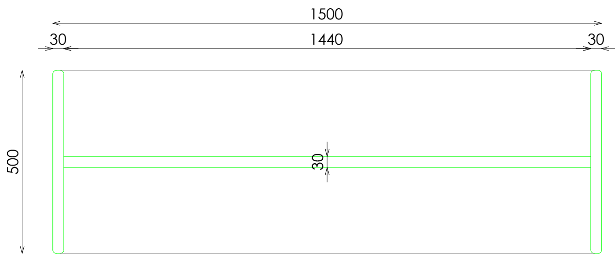
PLANTA SECCIONADA
