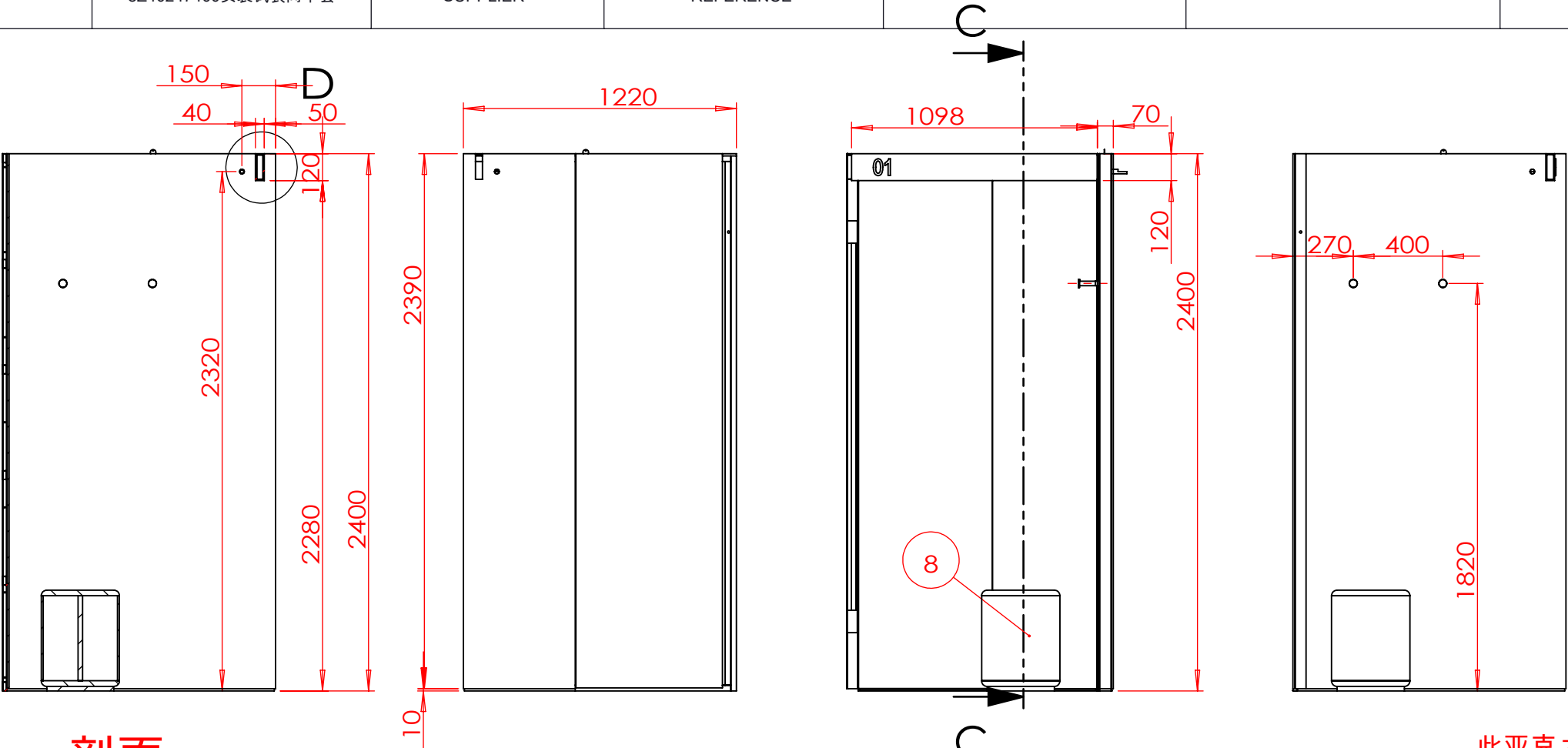
剖面 C-C
