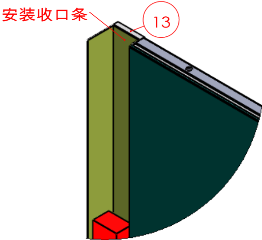
局部视图 E
