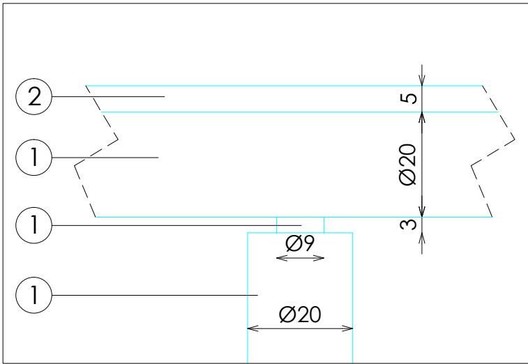
DETALLE B
