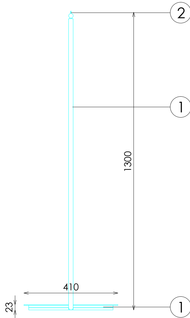
PERFIL
