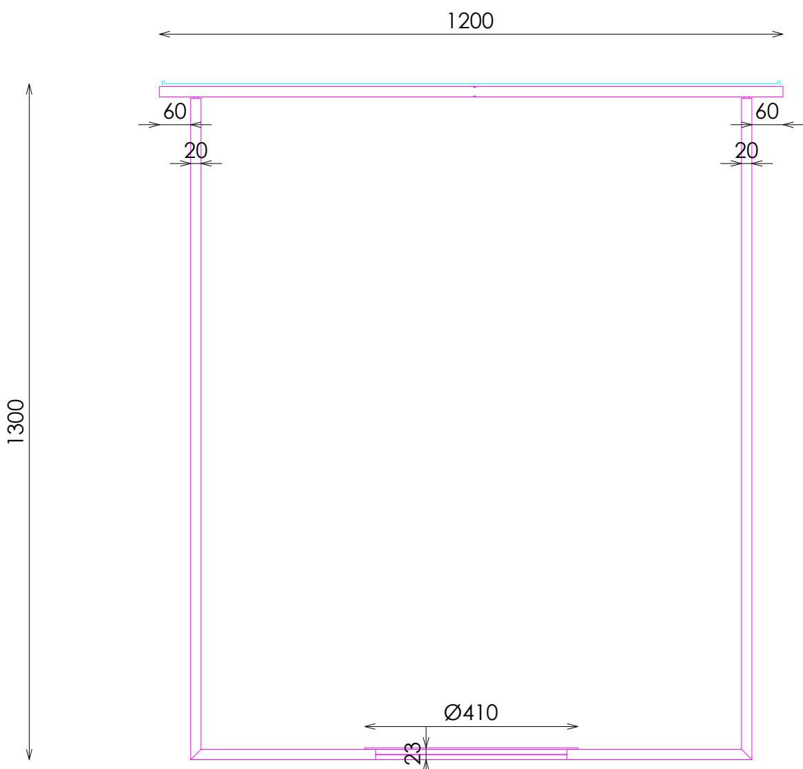
ALZADO
