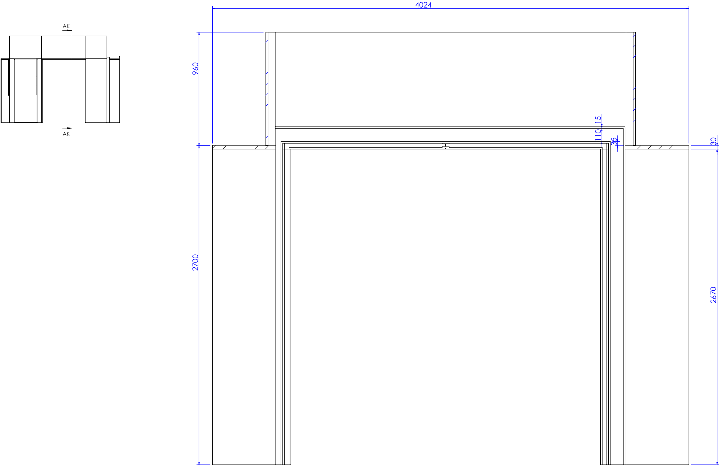
剖面 AK-AK 比例 1 : 20
