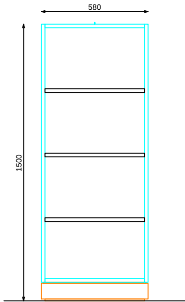
ALZADO LATERAL
