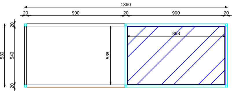
PLANTA SECCIONADA
