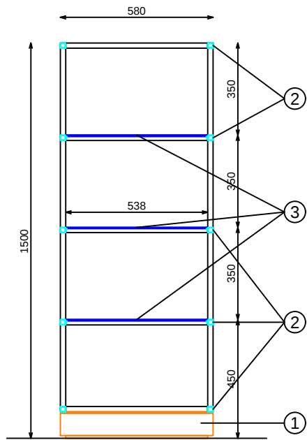
SECCIÓN BALDAS
