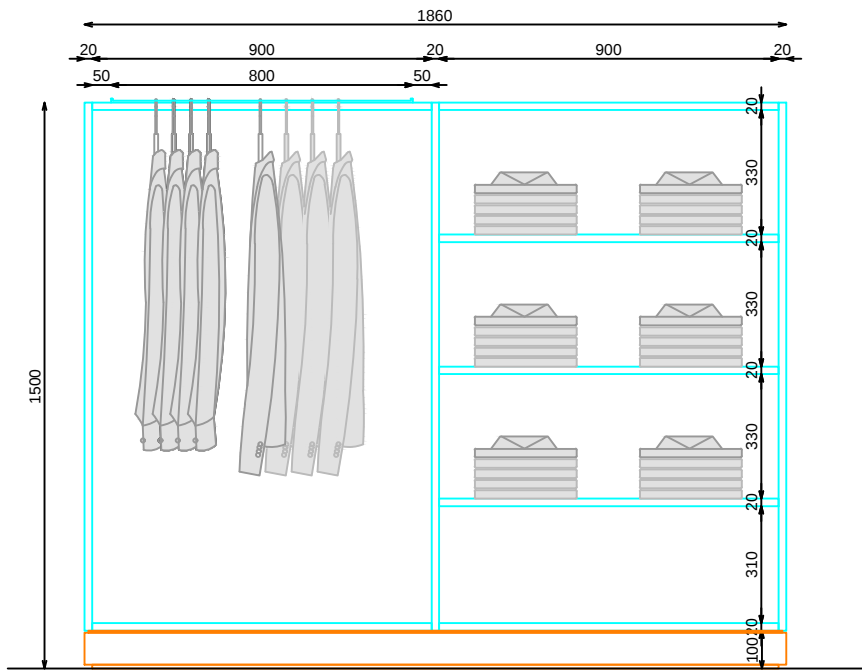
ALZADO FRONTAL
