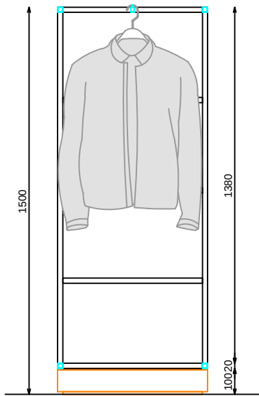
SECCIÓN CUELGA
