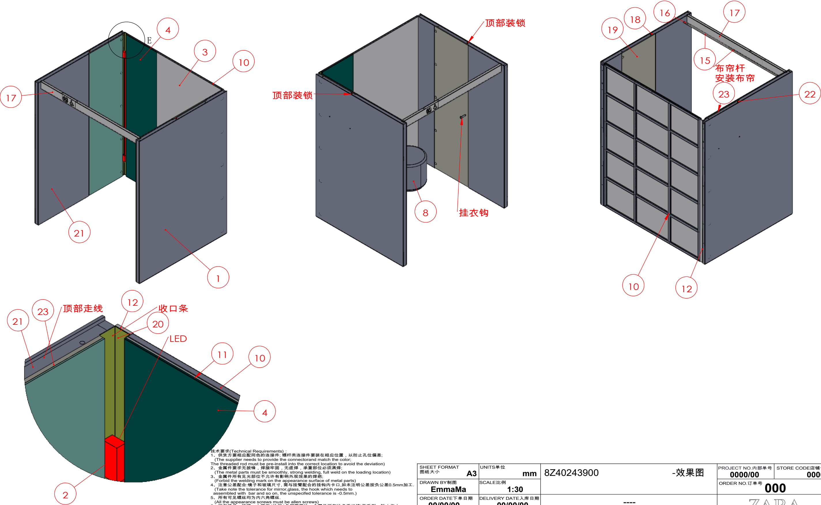
局部视图 E 比例 1 : 5
