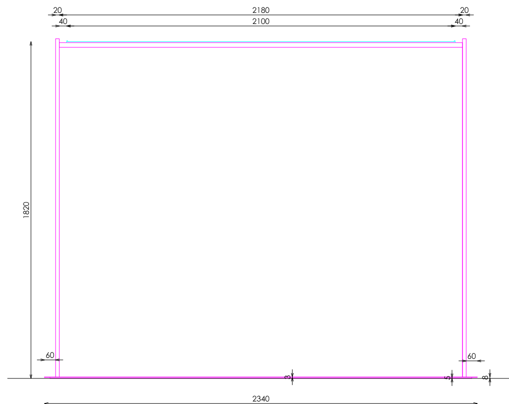
ALZADO SECCIONADO
