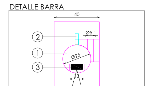
DETALLE EXTREMO BARRA
