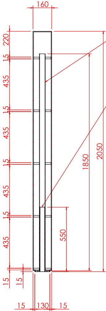
剖面 AH-AH
