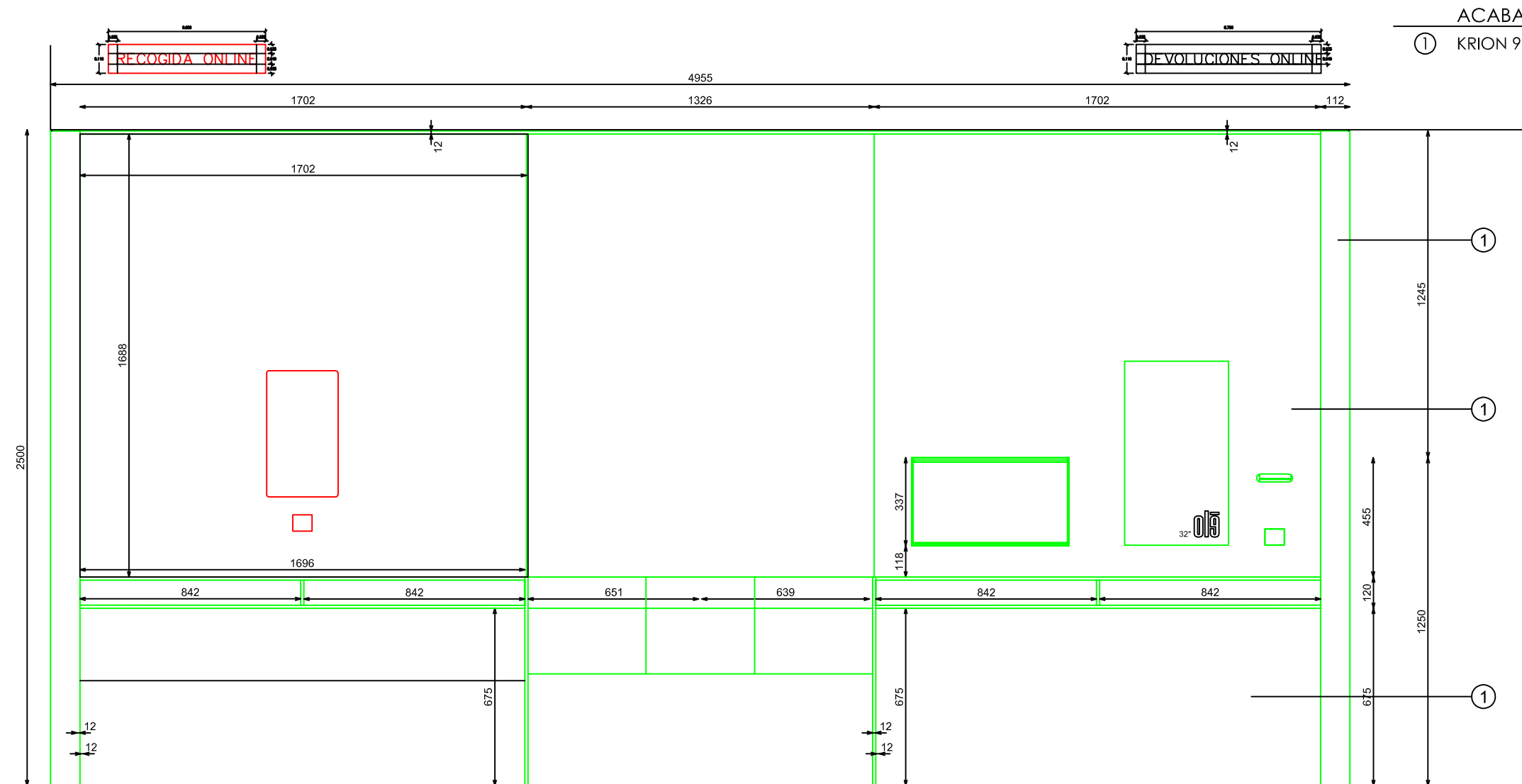
ALZADO FRONTAL
