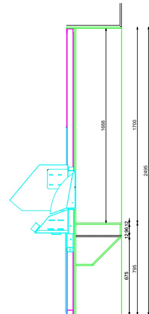
SECCION
