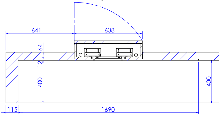
剖面 A-A
