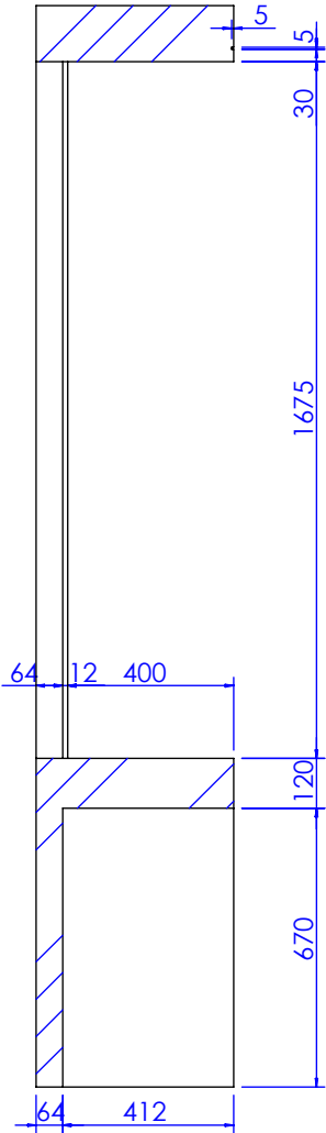
剖面 C-C
