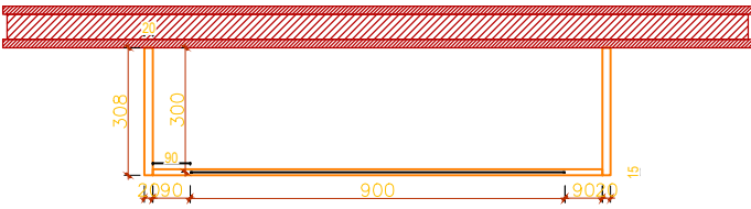
1 平面图 1:10 PLAN
