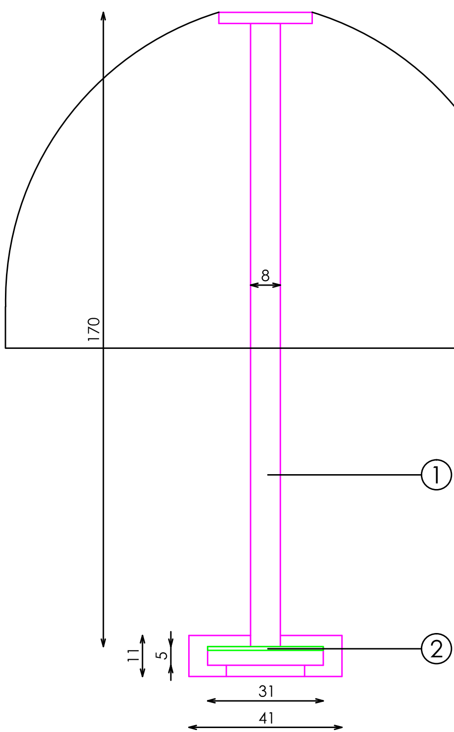
PERFIL
