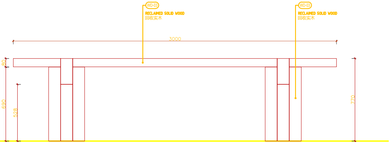
2 正立面 FRONT ELEVATION 1:10
