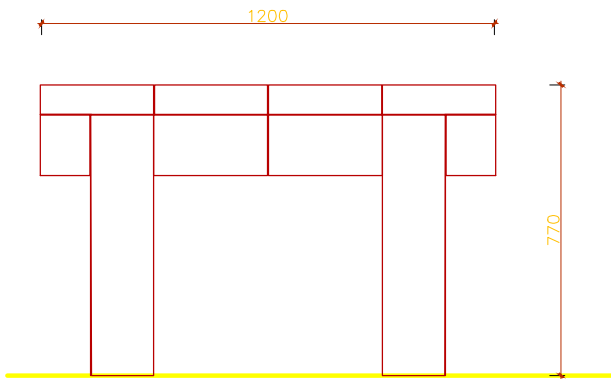
3 侧立面 SIDE ELEVATION 1:10
