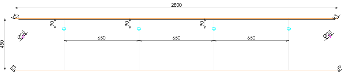
PLANTA TARIMA
