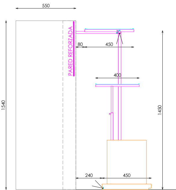
SECCIÓN
