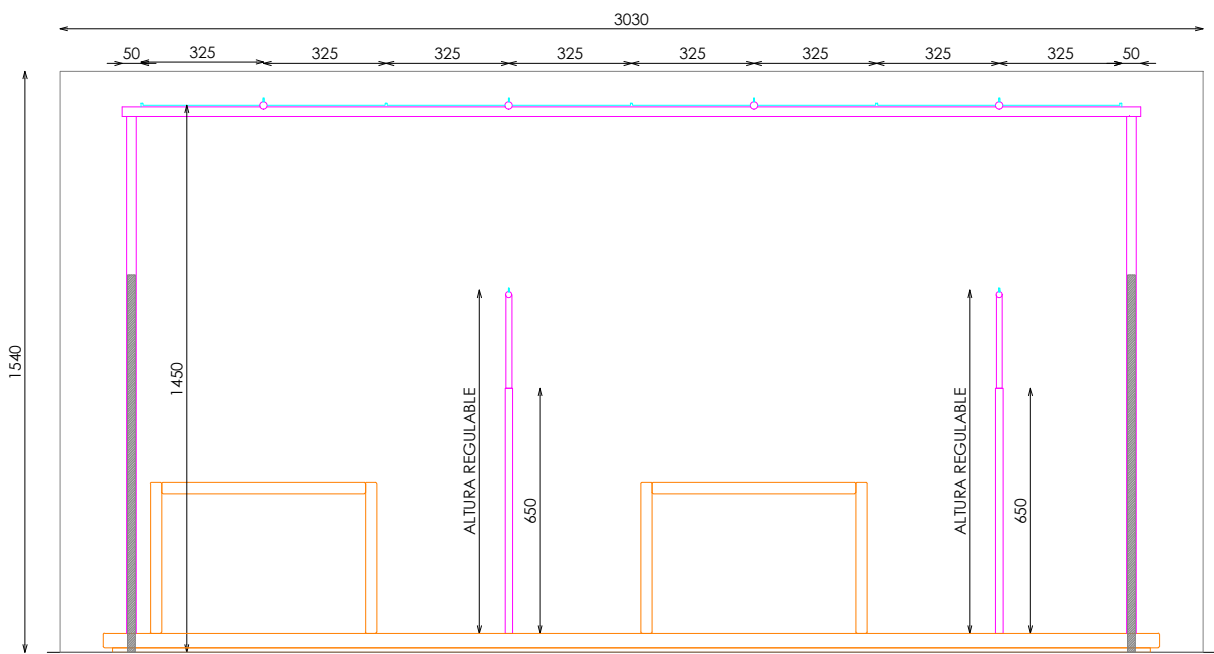
ALZADO FRONTAL
