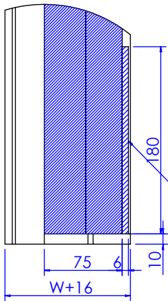
局部视图 AK 比例 1:5
