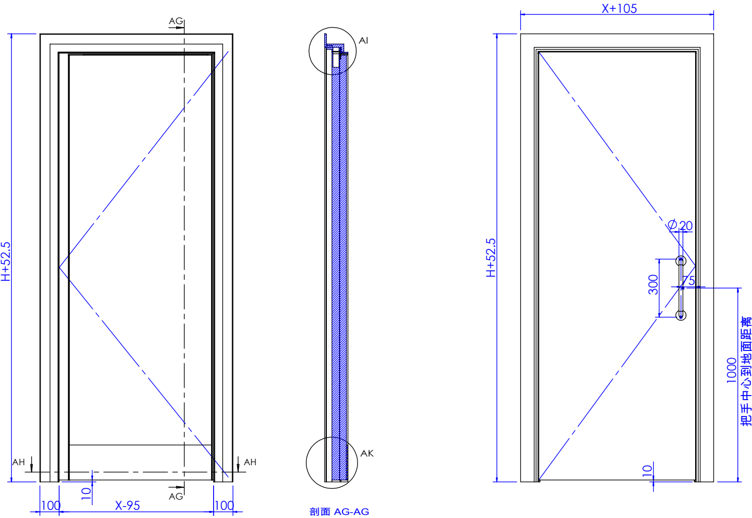
剖面 AG-AG
