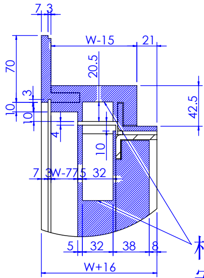
局部视图 AI 比例 1:4
